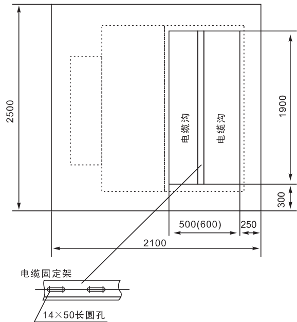
图4 预装式变电站建议台基尺寸图
