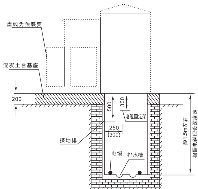
图3 建议台基尺寸
