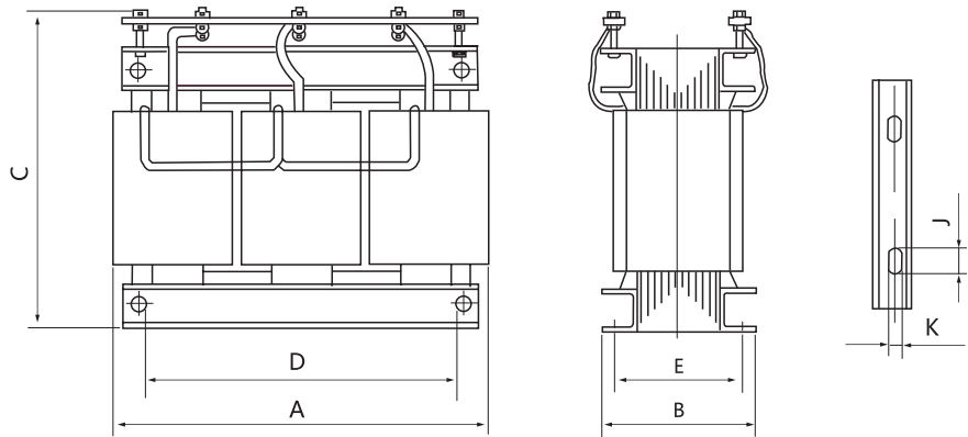
图1 开启式
