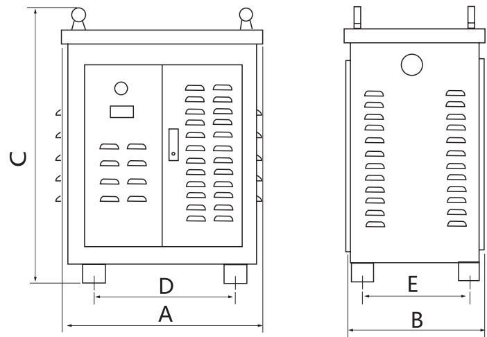
图3 防护式 30~130kVA
