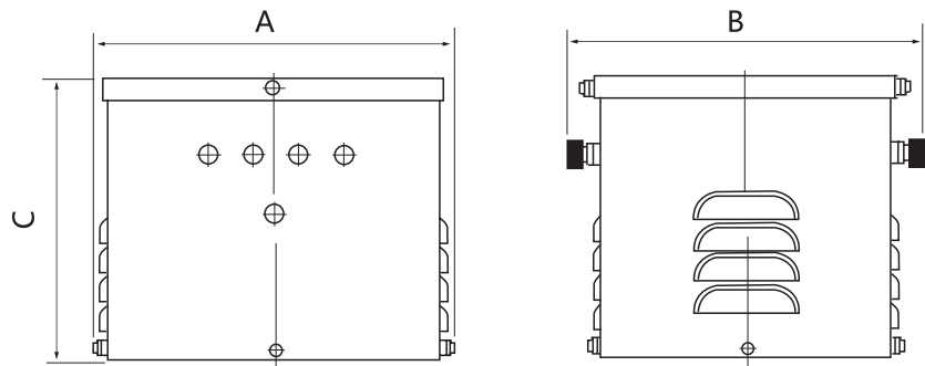
图2 防护式 0.5~20kVA
