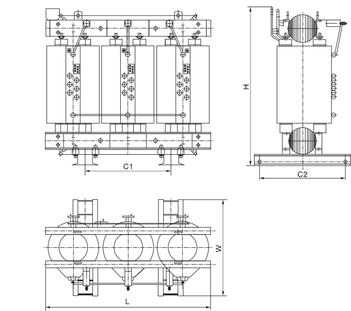
图1 SC(B)10-50-6300/35kV变压器外形及安装尺寸
