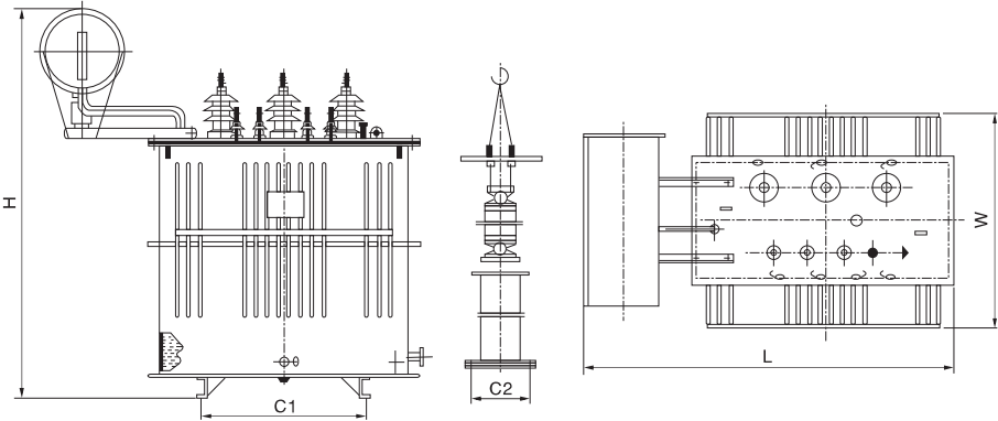
图1 S11-10 ~ 2000/10变压器外形及安装尺寸
