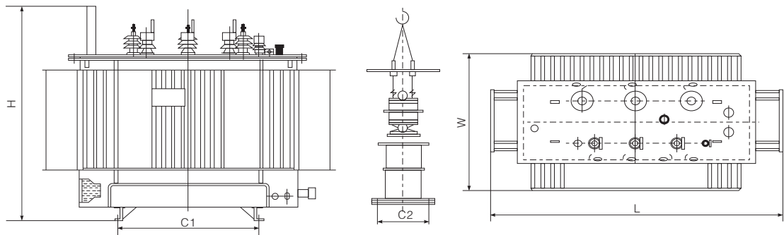
• 安装尺寸 表2
