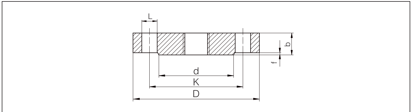
Fig. 8: Dimensions - EN flange EN 1092-1 (seal ledge B1)
